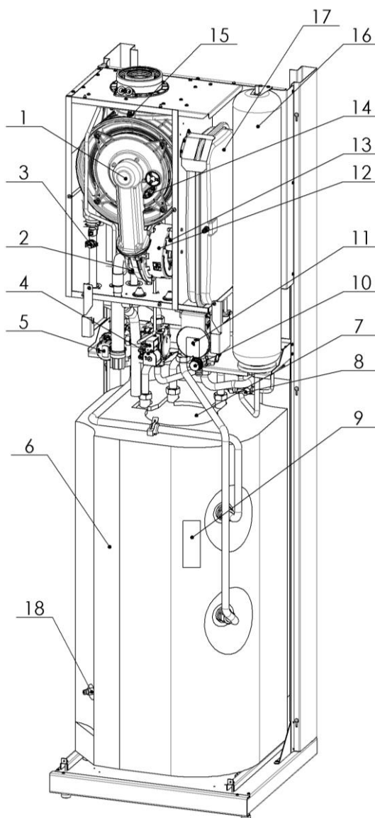
Rys.2.2.1.1. Rozłożenie elementów w kotle
