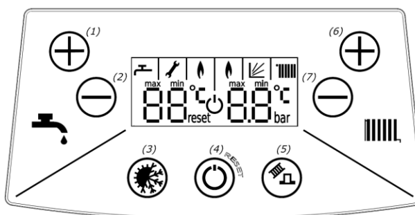
Rys. 5.2.1. Panel sterowania
