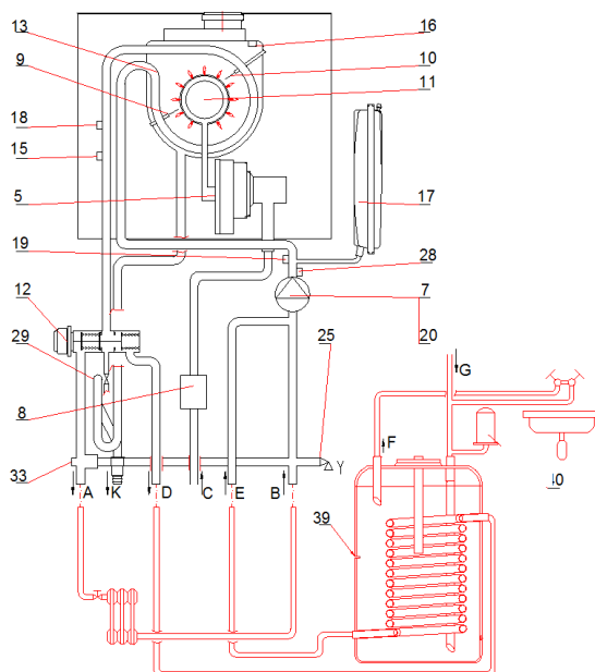
Rys.2.2.1.2. Schemat ideowy
